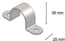
T1-Buisklem RVS | Ø40/38 mm, 25 x 2 mm
